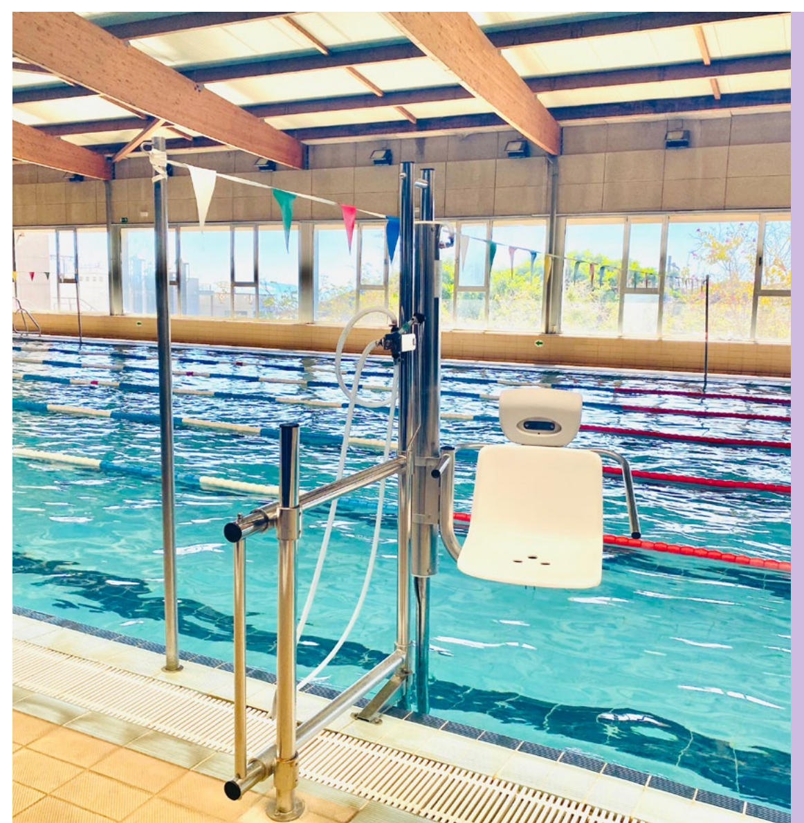
Grúa piscina
